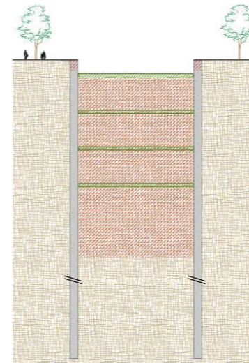
Phase 3 : Recépage 7 des parois moulées, terrassement à ciel ouvert et pose progressive des butons provisoires
