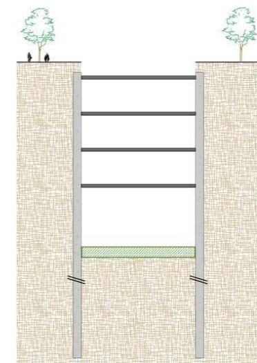
Phase 4 : Réalisation du radier
