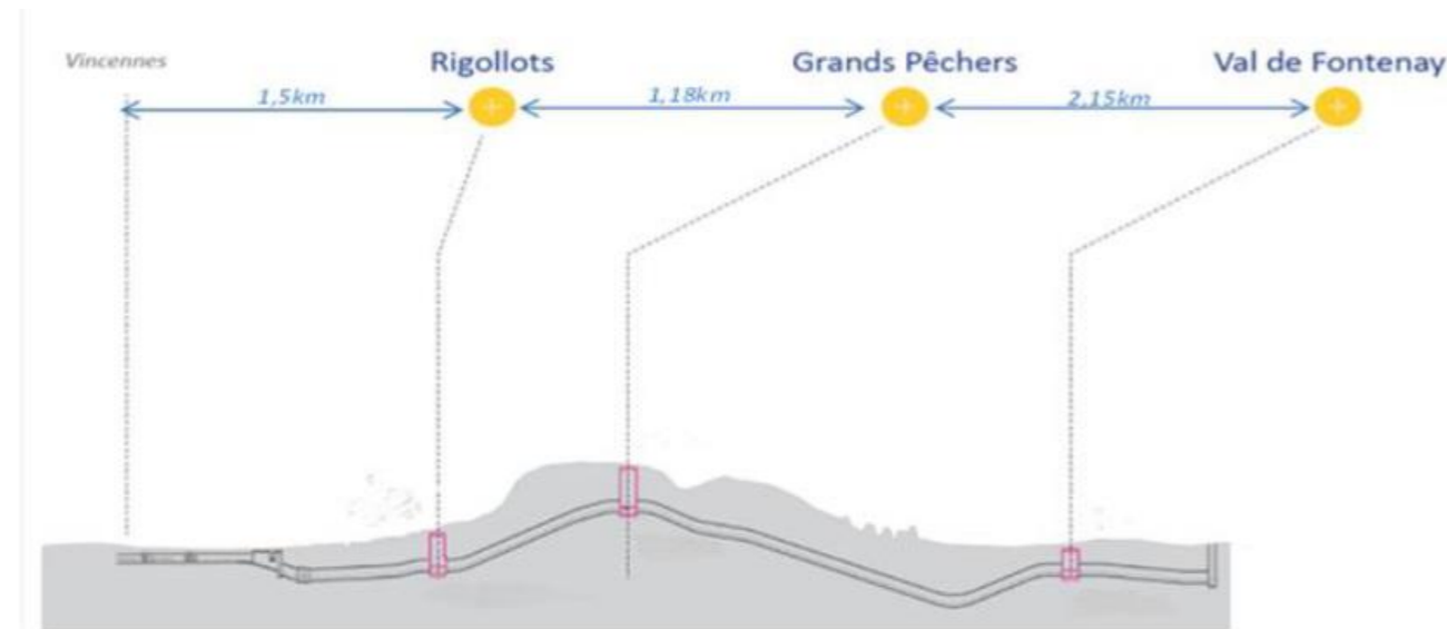
Figure 43 – Profil en long (Source : Agence Véra Broëz)
