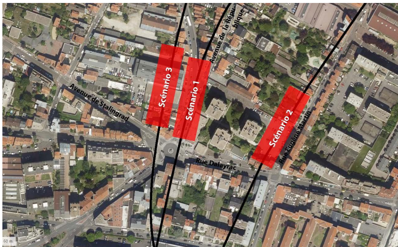
Figure 40 – Variantes d'implantation de la station Les Rigollots (Source : Ingérop)
