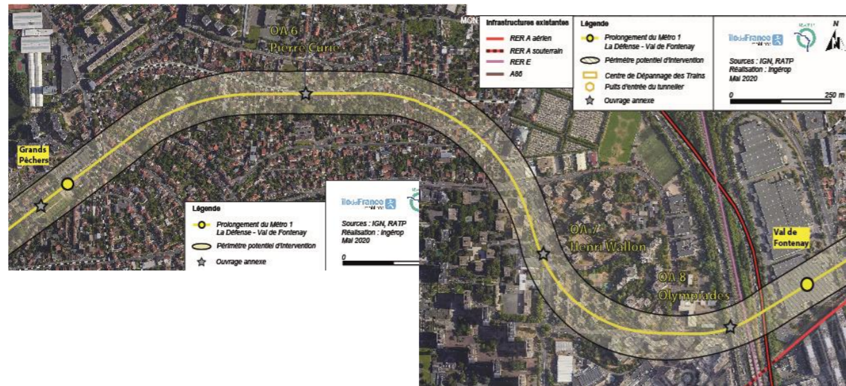
Figure 49 – Extrait du PGT – Zoom entre les stations Grands Pêcheurs et Val de Fontenay (Source : Ingérop)
