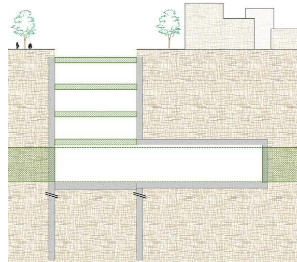
Phase 6 : Passage du tunnelier puis réalisation des dalles intermédiaires et enlèvement des butons provisoires
