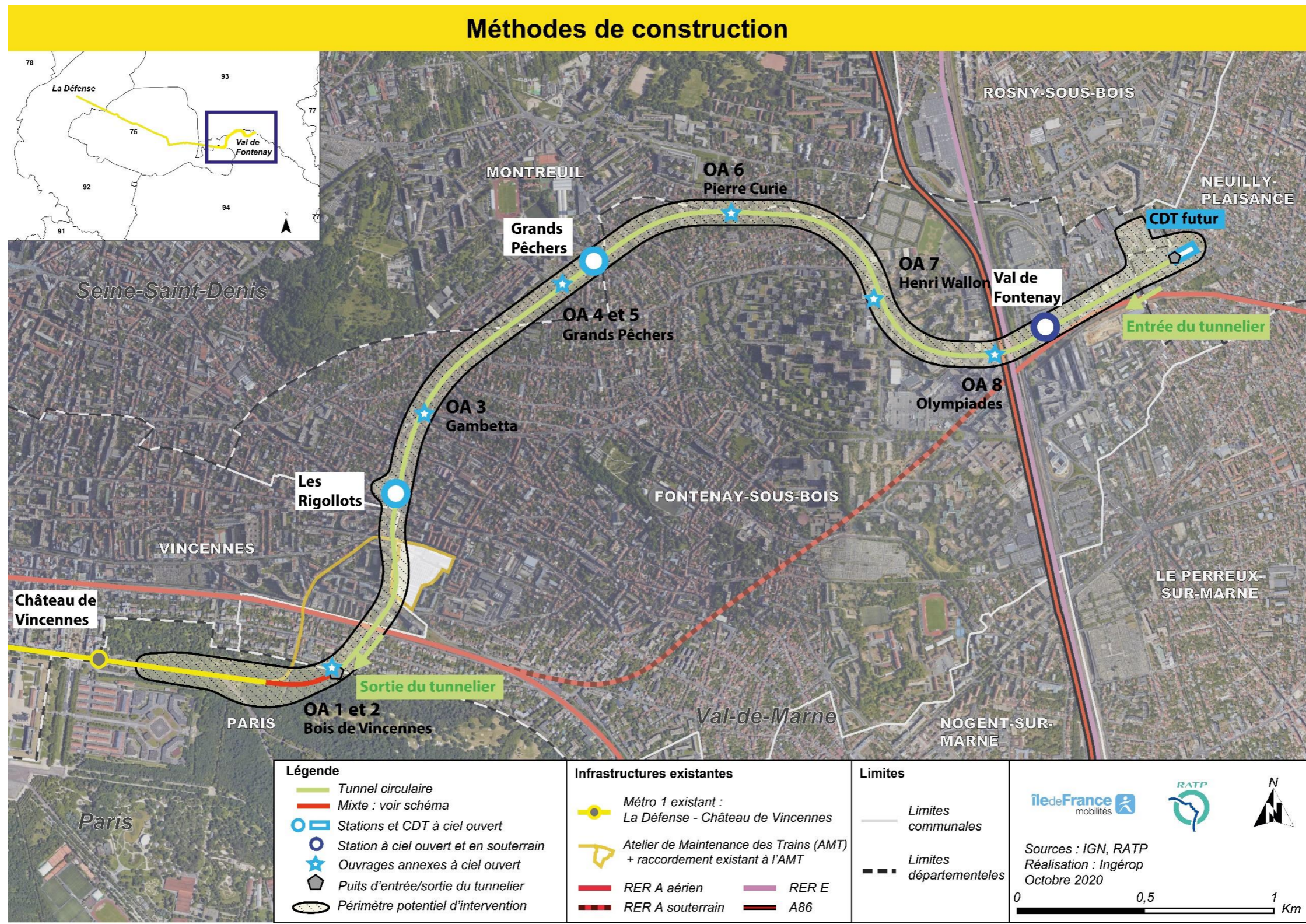
Figure 83 – Synthèse des méthodes constructives envisagées pour la réalisation des ouvrages constitutifs de l'opération (Sources : RATP – Ingérop)
