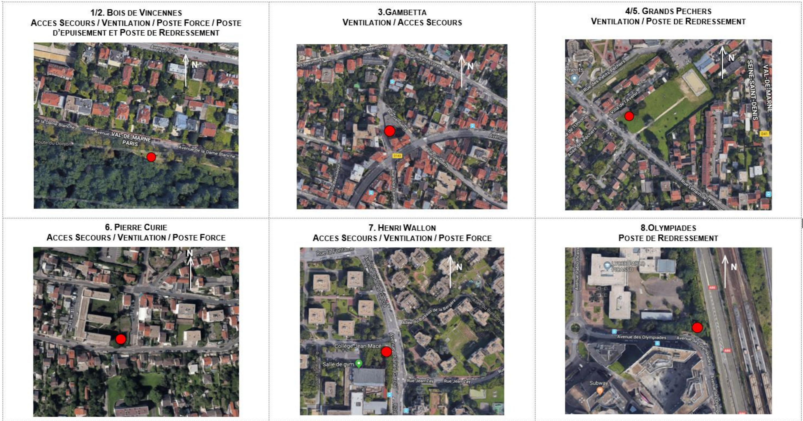
Figure 77 – Localisation indicative des ouvrages annexes (Source : Etudes préliminaires RATP)
