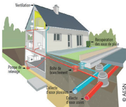
Fonctionnement du réseau séparatif
